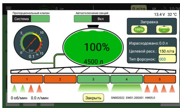
В данном примере включены: 3 и 4 секции, 4 управляемые форсунки на 5 секции и 2 управляемые форсунки на 1 секции.
